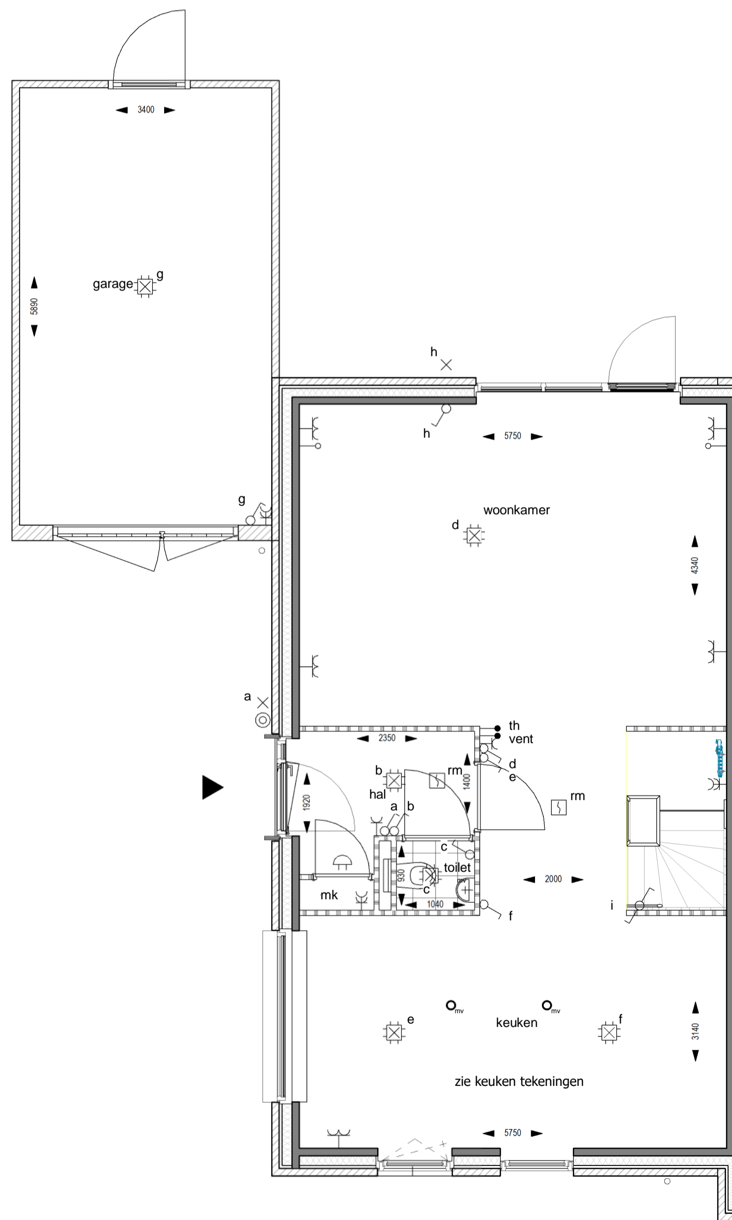
Begane grond
