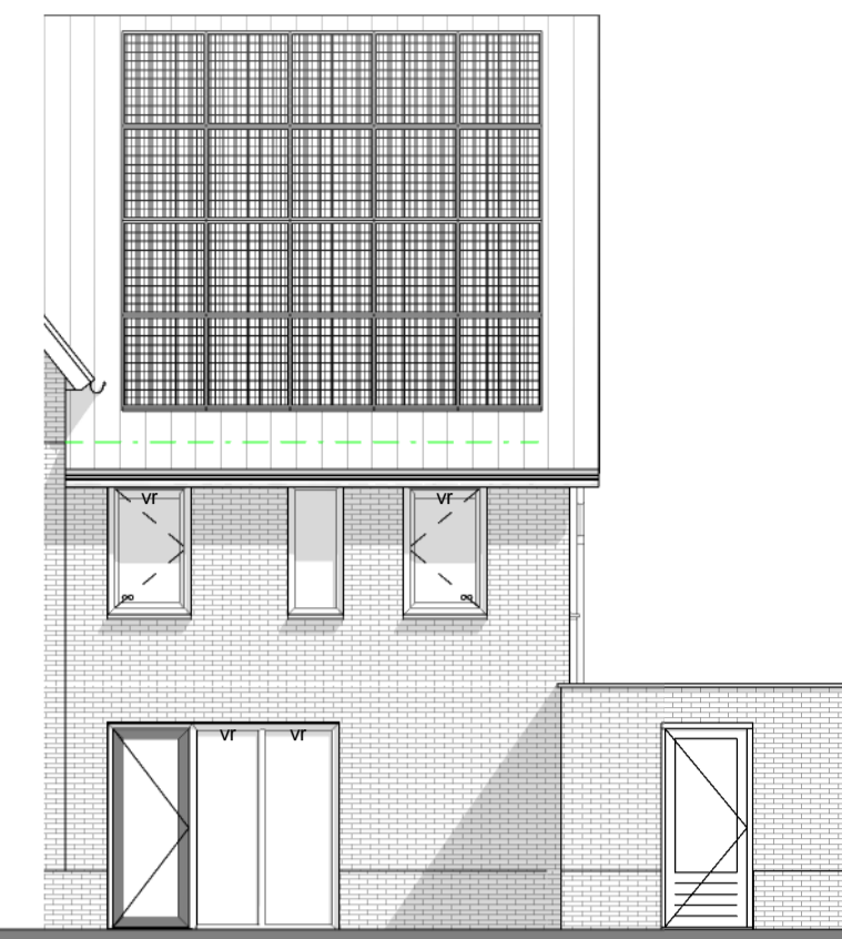
Achtergevel
