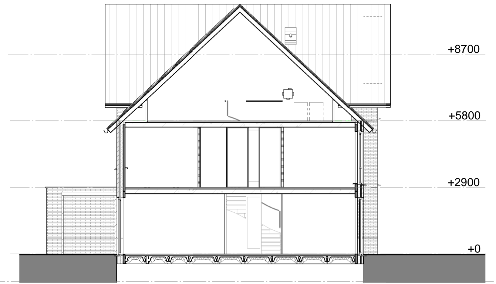
Doorsnede C
