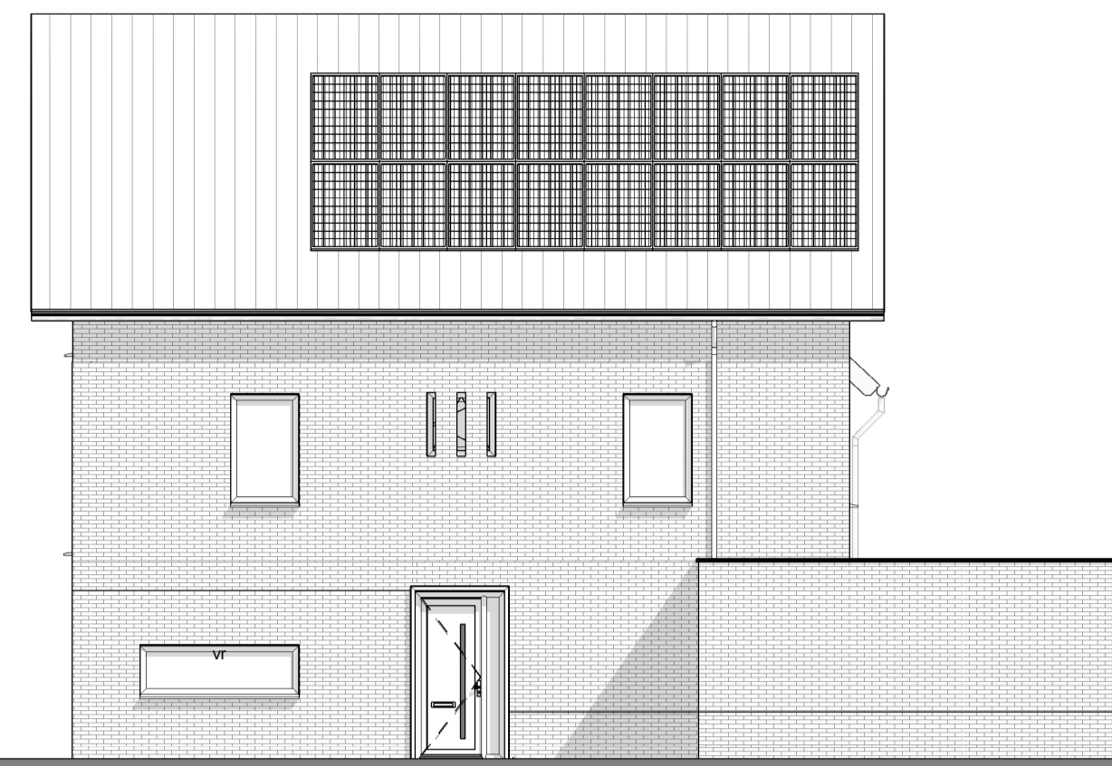
Rechtergevel - Blok 4
