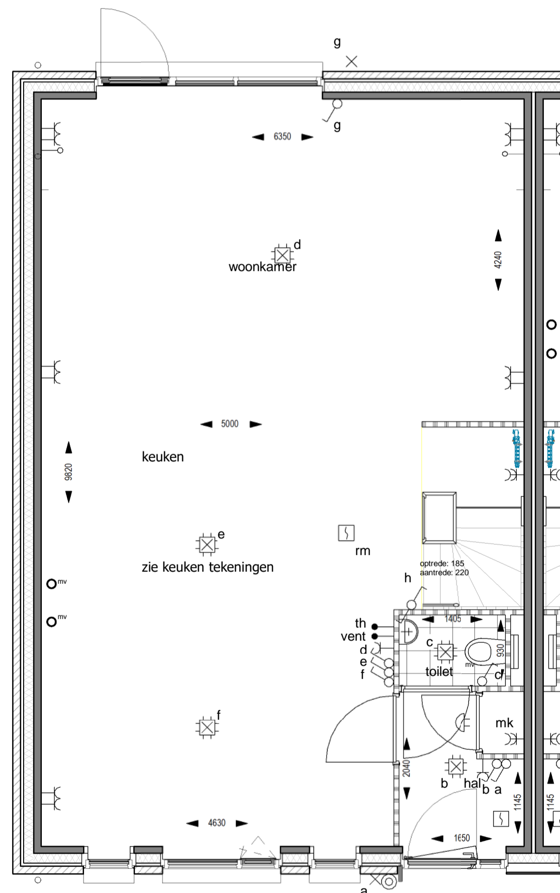
Begane grond
