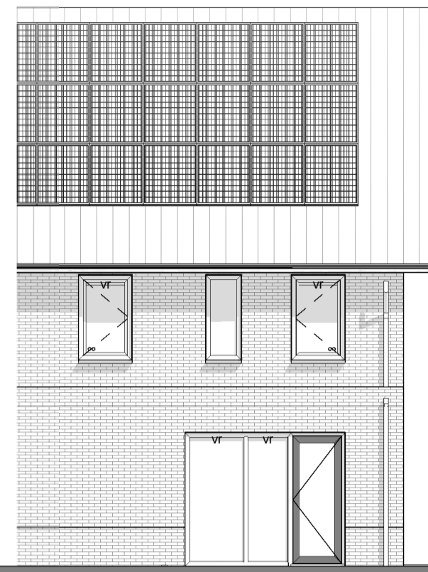
Achtergevel
