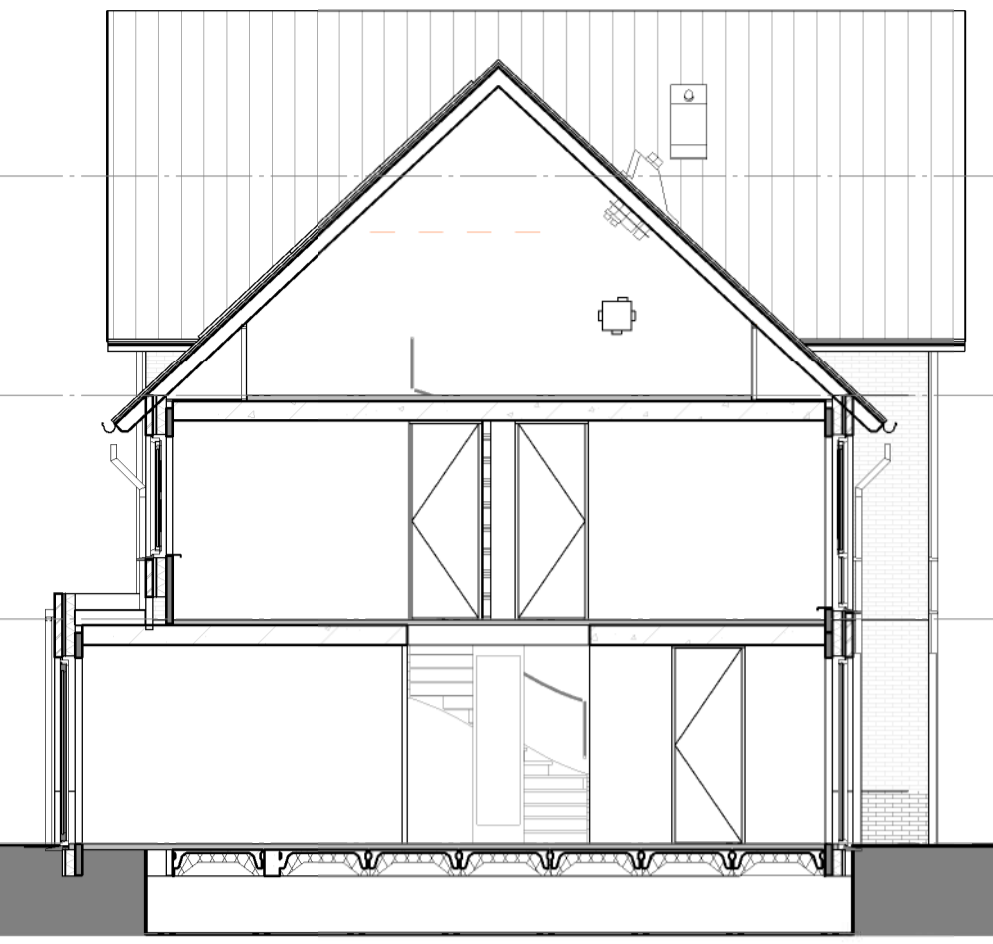
Doorsnede C
