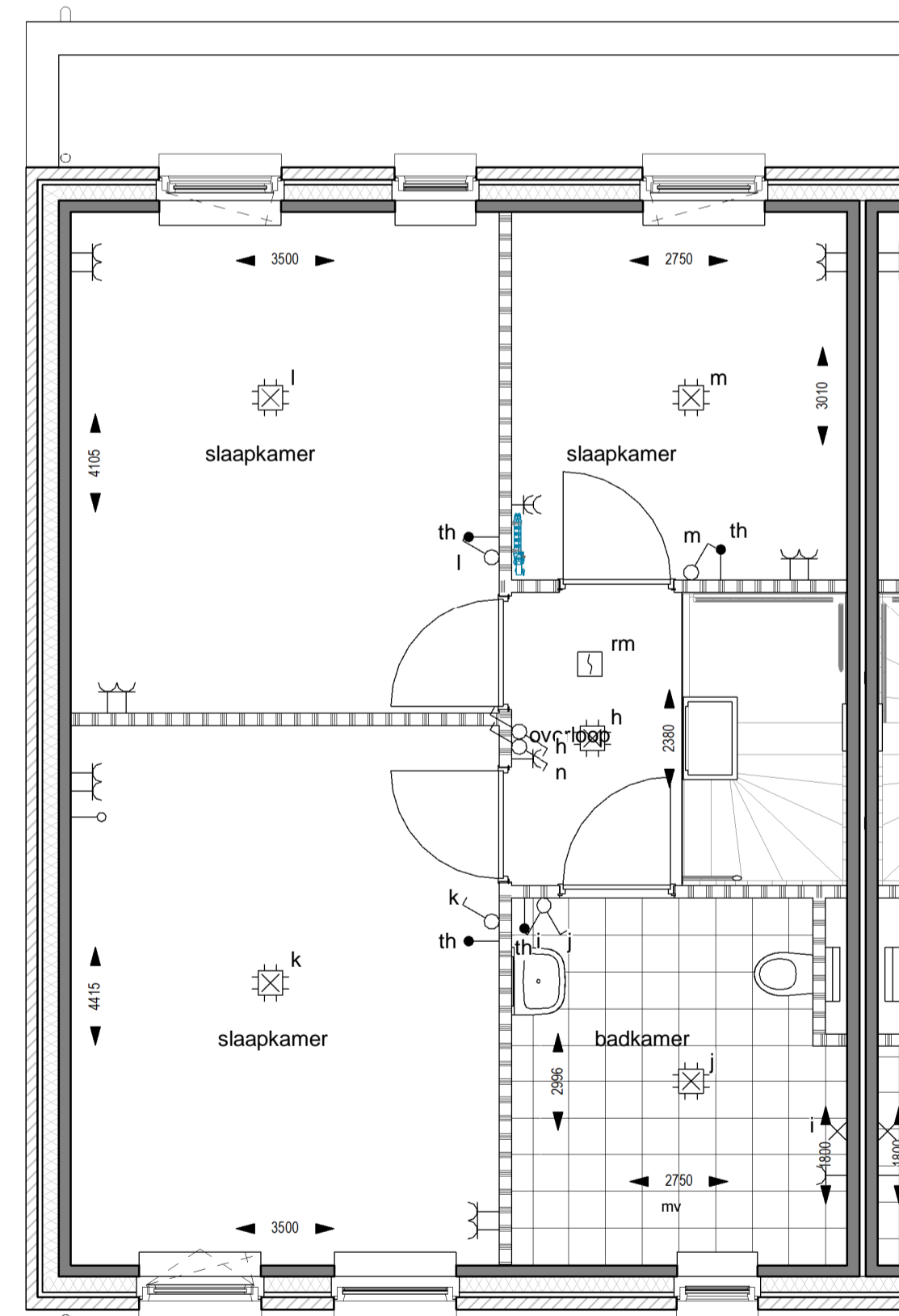
Verdieping 1
