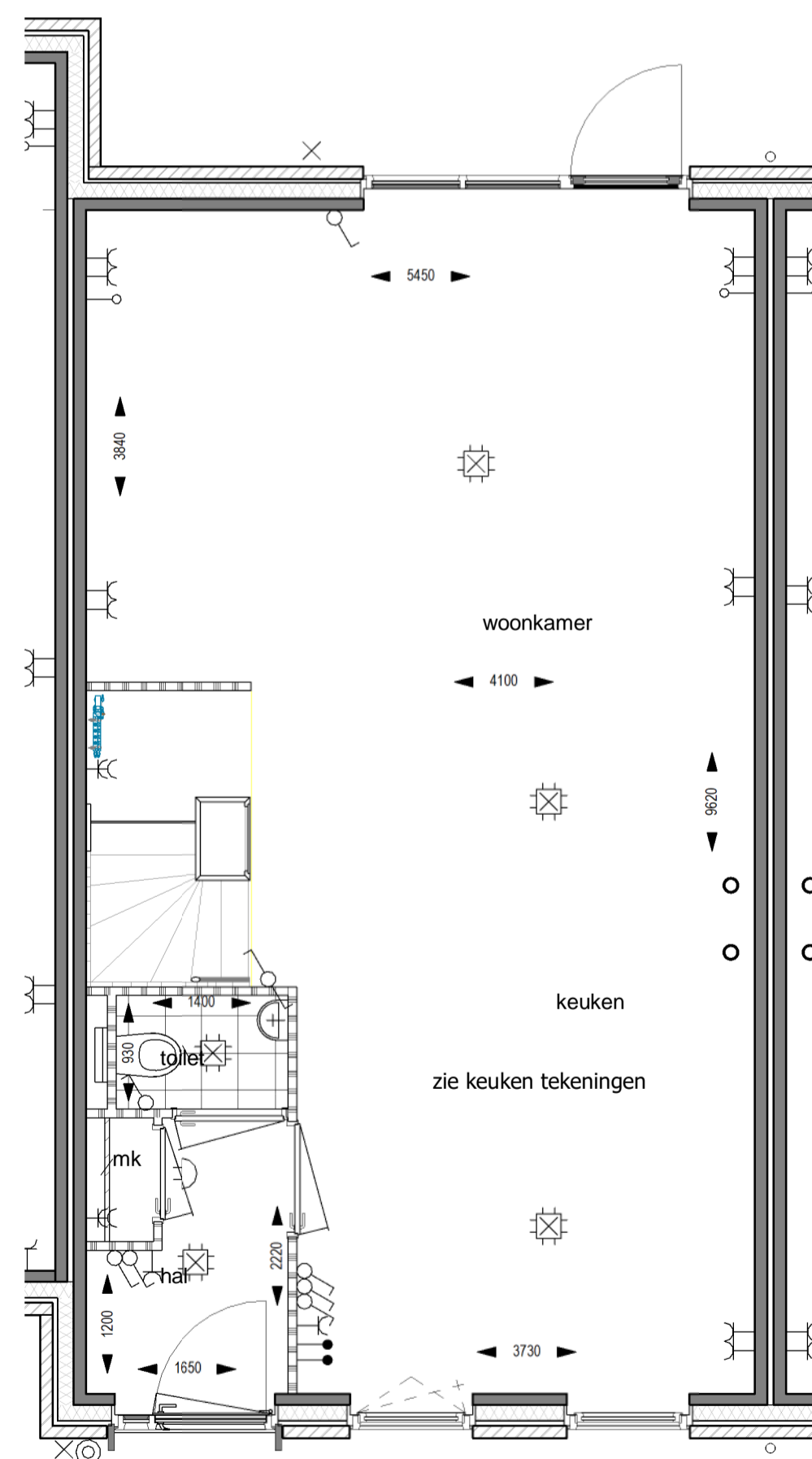
Begane grond
