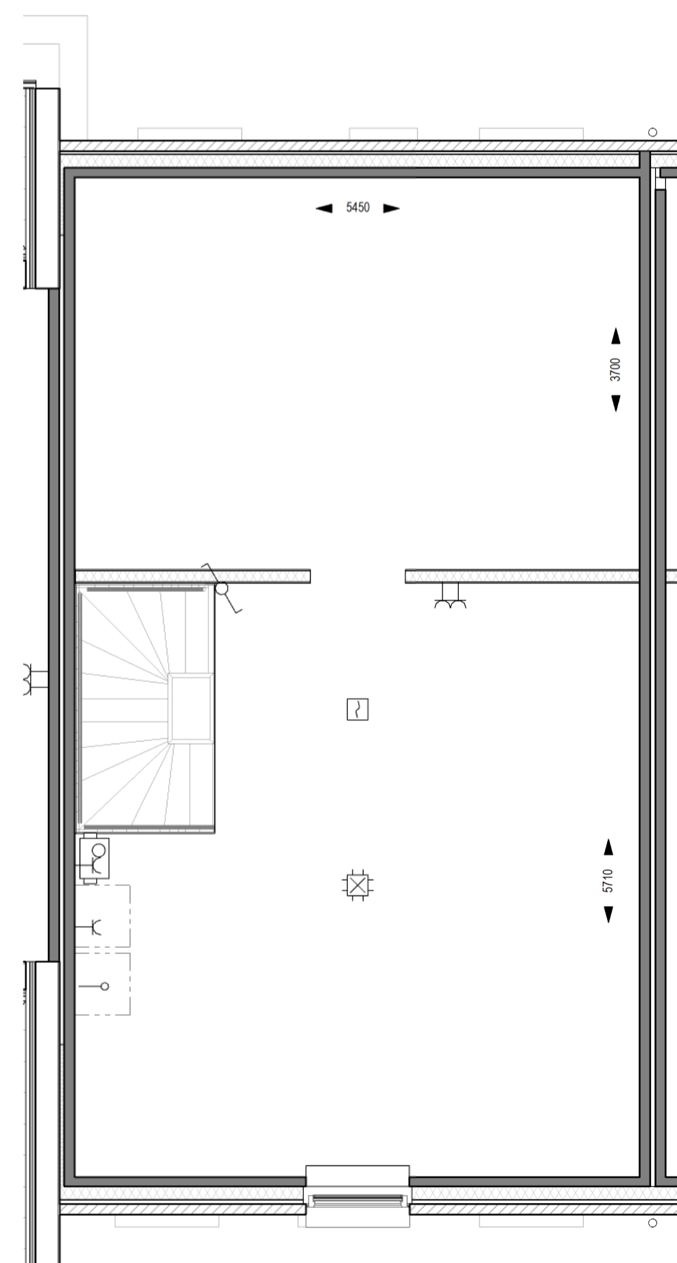
Verdieping 2
