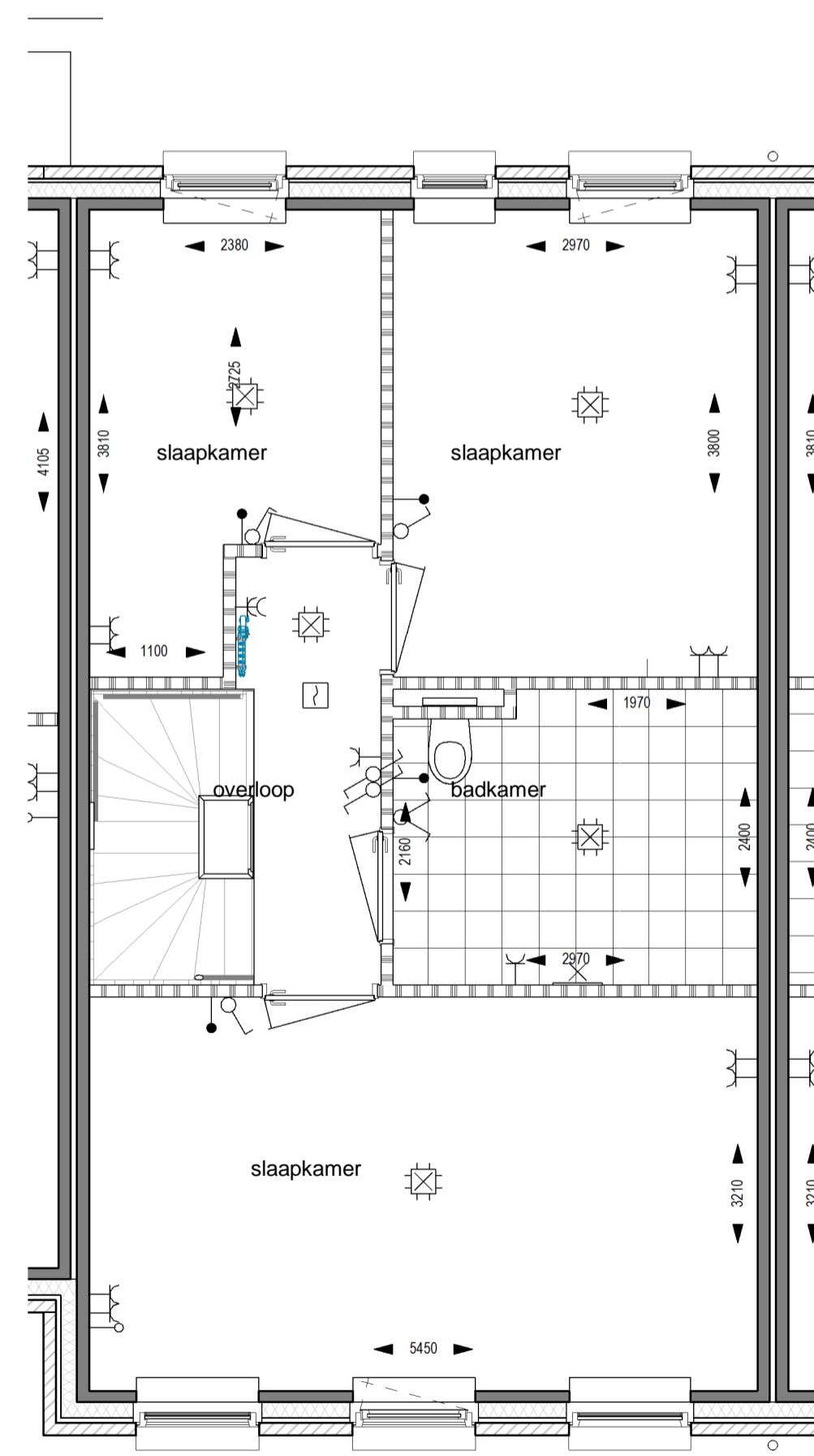
Verdieping 1
