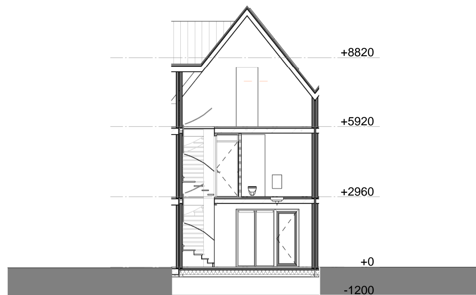
Doorsnede
