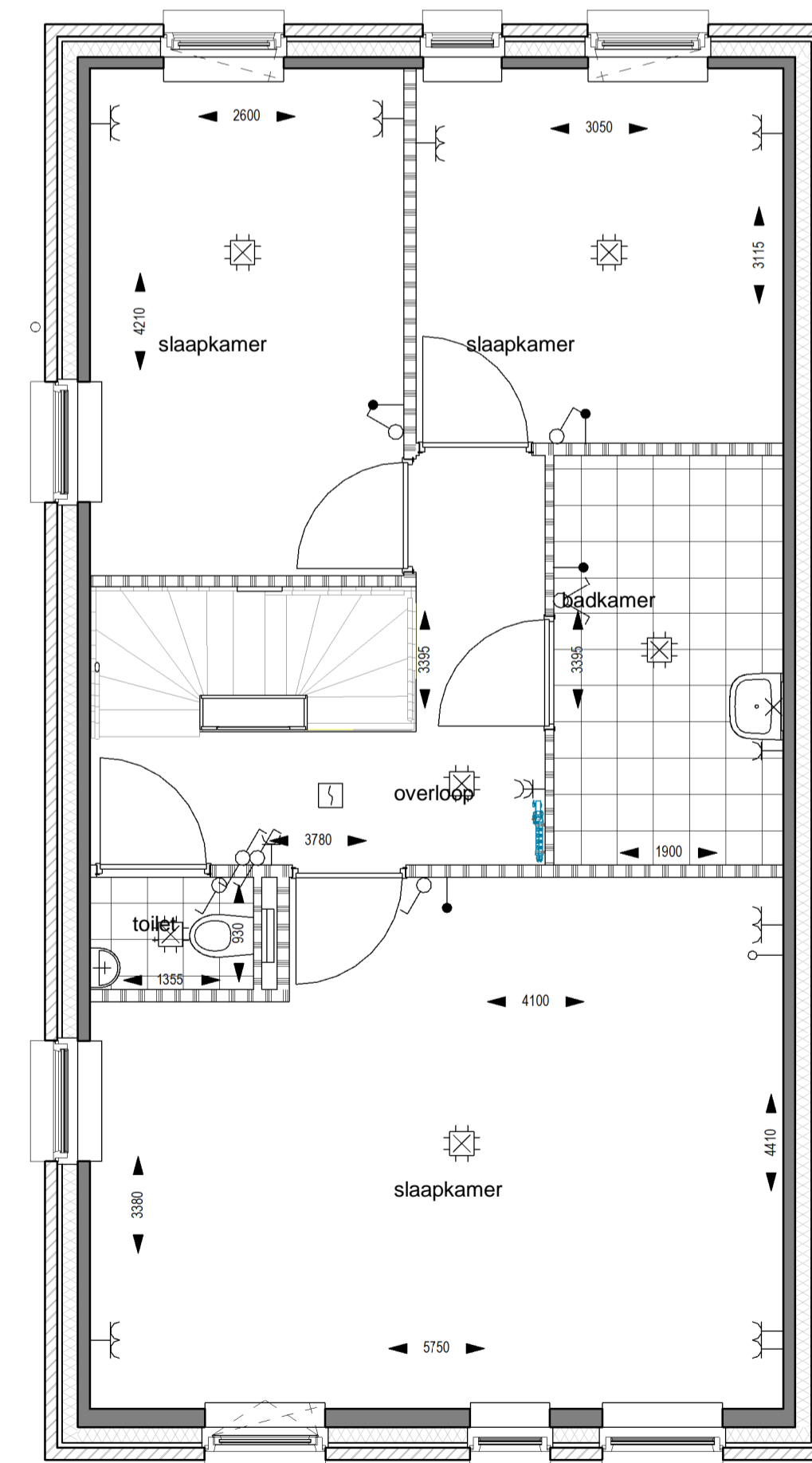
Verdieping 1
